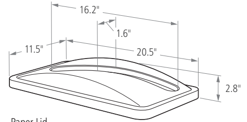
Paper Lid
